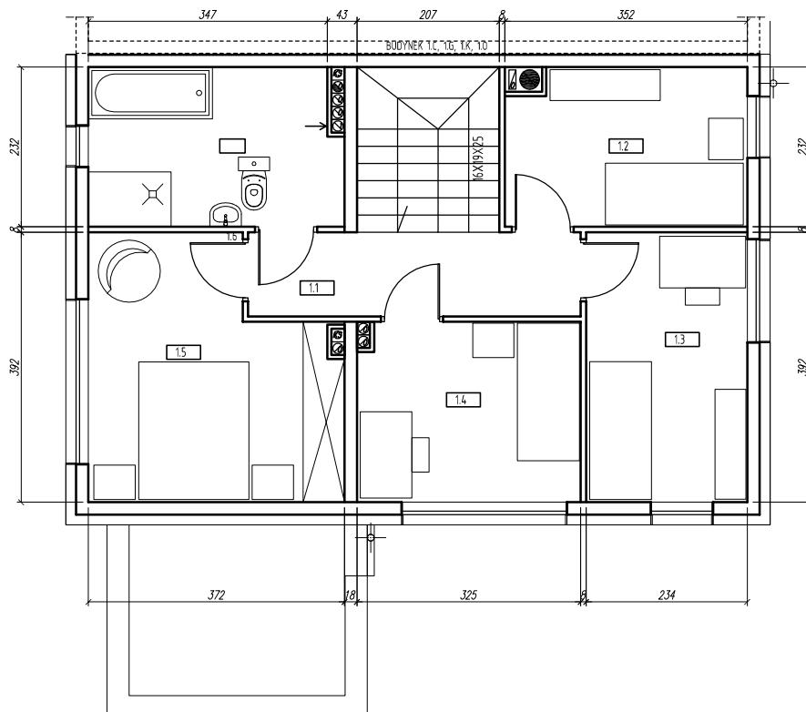
PIĘTRO SKALA 1:100
